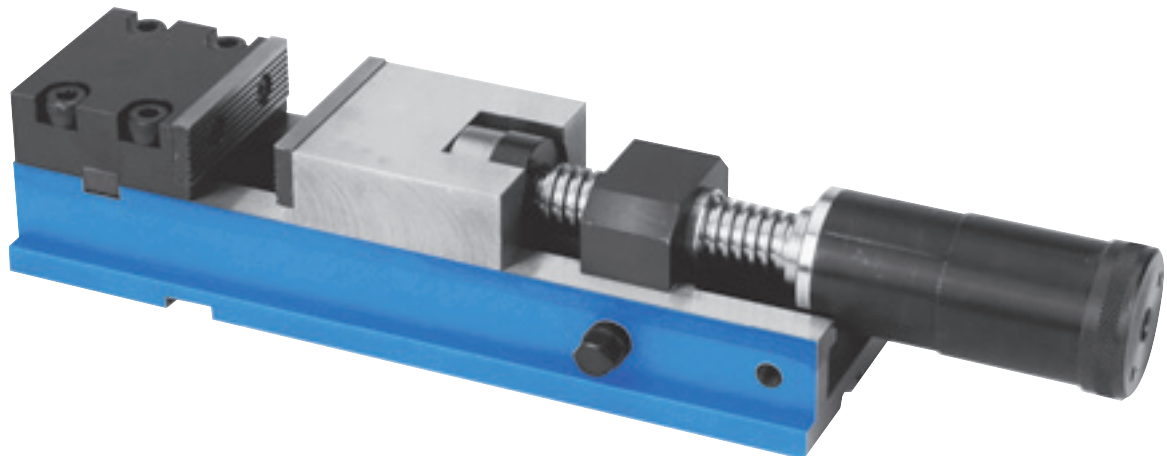
KORNA RASANT mit pneumohydraulischem Spannsystem
